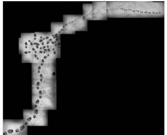
Alessandro Scali e Robin Goode, Oltre le colonne d'Ercole, 2006, silicio con strato di ossido cresciuto termicamente, litografia ottica con resist positivo, attacco chimico in HF, supporto mm 10x10, impronta più piccola um 135x460, immagine FESEM (Field Effect Scanning Electron Microscope).
